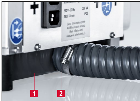
Figure 7-22 Réservoir à déchets avec embout d'aspiration
