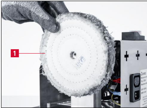
Figure 7-20 Remplacement du disque de polissage
