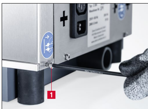
Figure 7-15 Desserrer le capot du disque de polissage
