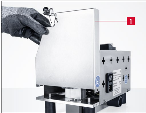
Figure 7-17 Retirer le capot du disque de polissage
