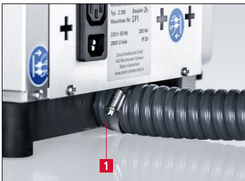
Figure 3-4 Bac à déchets avec embout d'aspiration
