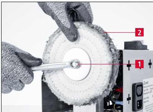
Figure 7-18 Desserrer le disque de polissage
