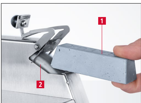
Figure 7-7 Appliquer la pâte à polir
