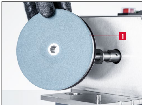
Figure 7-13 Retirer les disques d'affûtage usés
