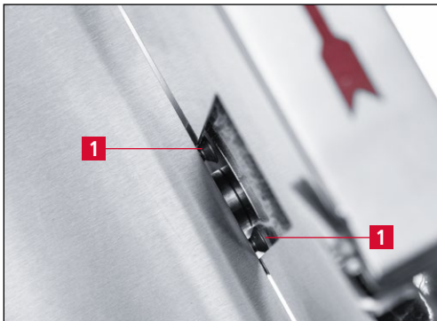
Figure 7-21 Vis de positionnement du capot du disque de polissage
