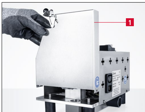
Bild 7-17 Polierscheibenabdeckung abnehmen
